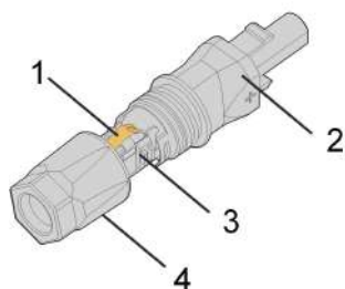
Rys. 4-1 Elementy złącza SUNCLIX
