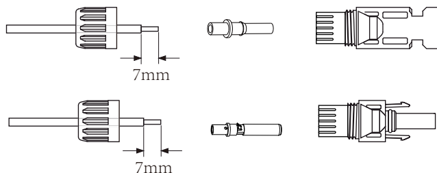
Rys. 3.3 Zdemonstuj nakrętkę kołpaka złącza
